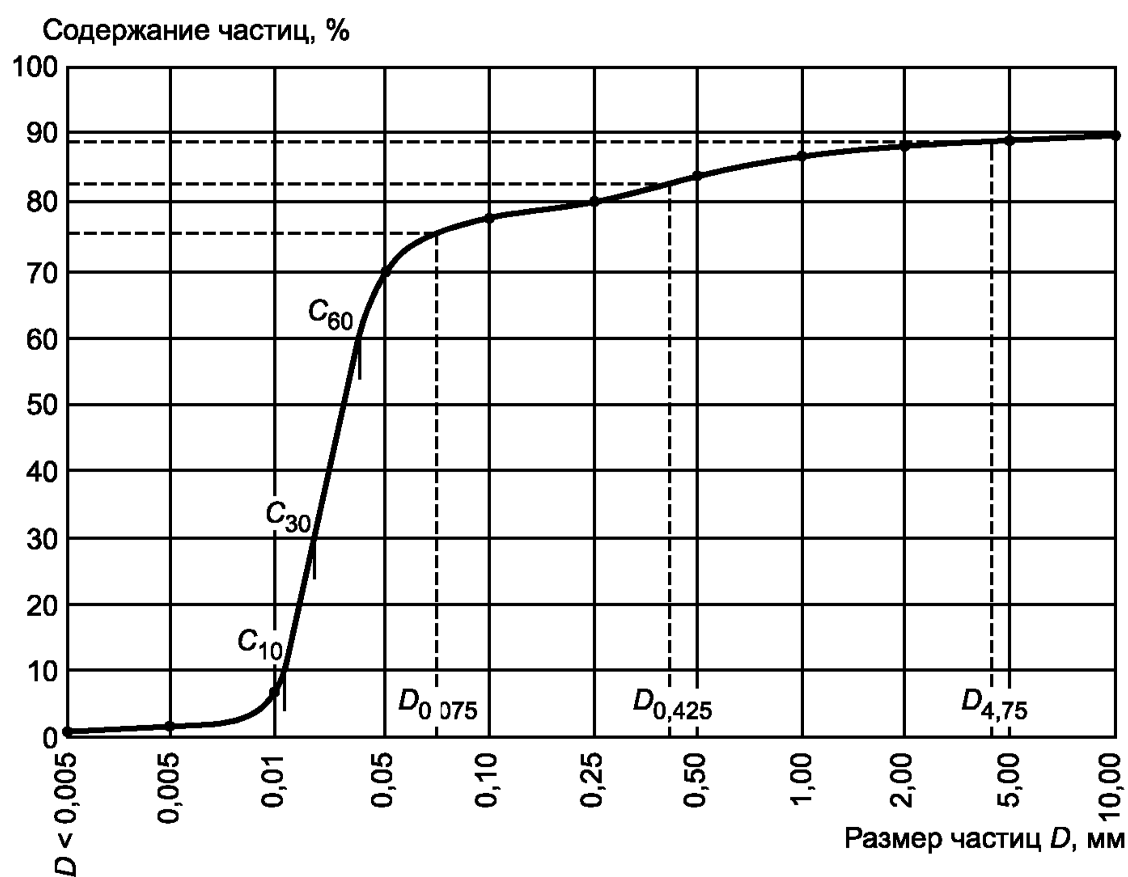
Рисунок Е.2 — Кумулятивная кривая гранулометрического состава
